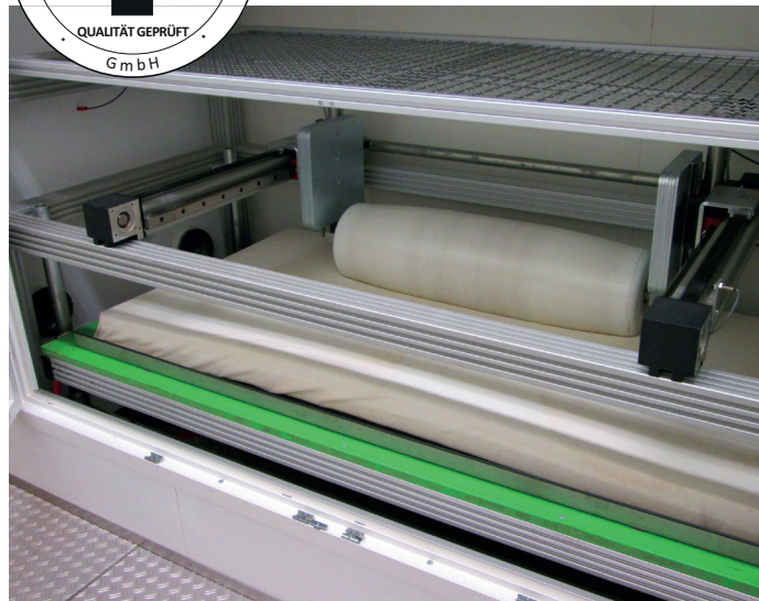
Prüfstand zur Funktionsprüfung von Matratzen Klima-Umhausung zur Prüfung unter speziellen Umgebungsbedingungen
